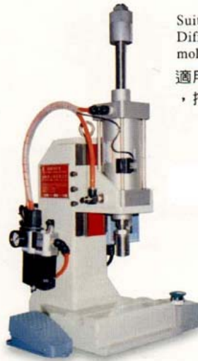
IDLE PRESSURE PRESS HC-300K 空壓壓床 MAX Power : 300 kg t/cm 2
